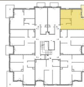
RZUT KONDYGNACJI
