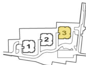
SCHEMAT OSIEDLA
