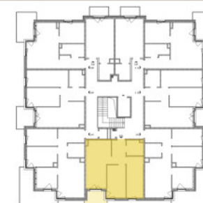
RZUT KONDYGNACJI
