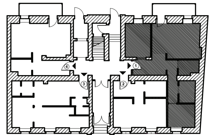
Rzut parteru skala 1:200
